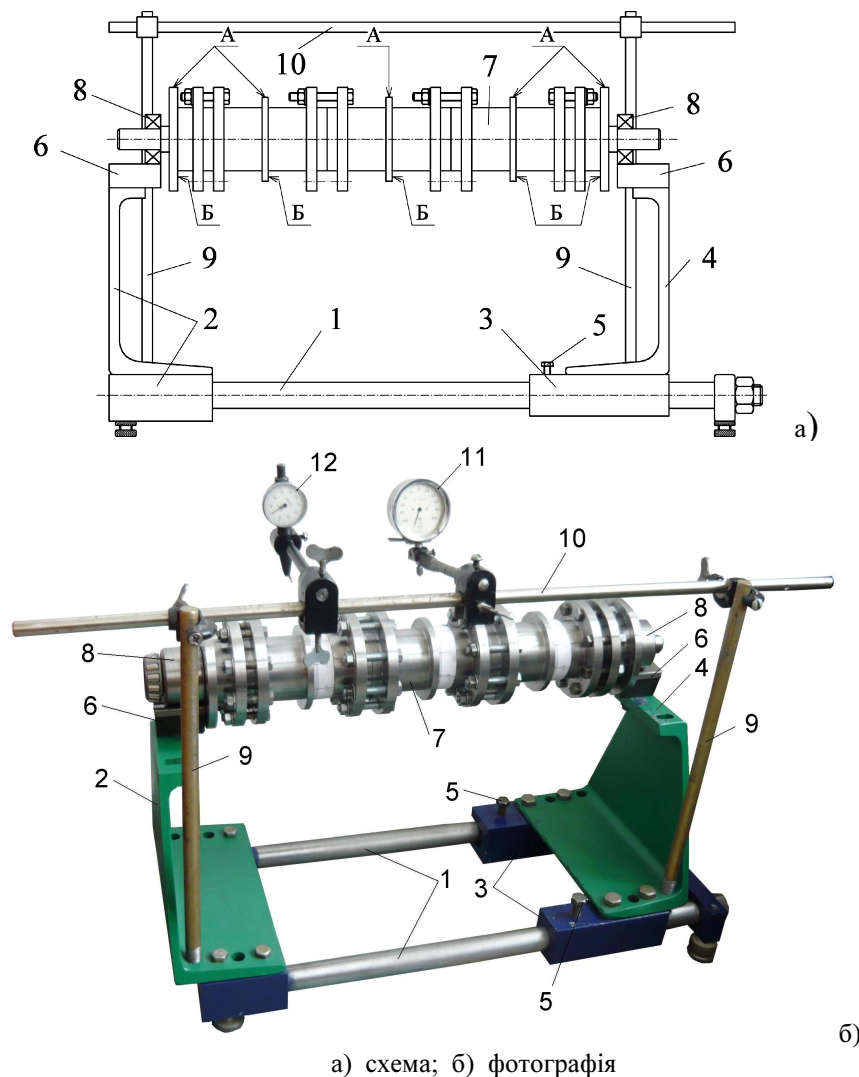
Рисунок 1 – Контрольне пристосування для встановлення міжопорного ротора на дві опори
