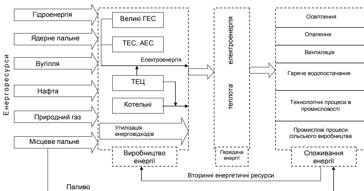
Рис. 4.1. Система централізованого енергопостачання промислових підприємств: ГЕС – гідроелектростанція; ТЕС – теплова електростанція; АЕС – атомна електростанція; ТЕЦ – теплоелектроцентраль
