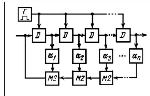
Рисунок 1 – Загальна схема регістра зсуву зі зворотнім зв'язком
