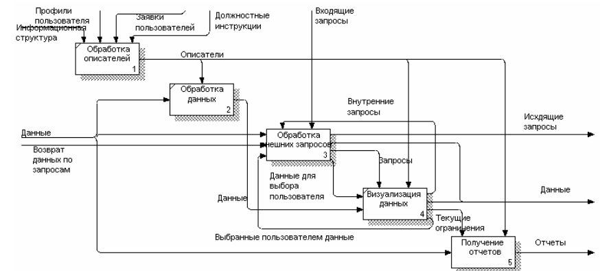
Рисунок 1 – Функціональна схема ТПК
