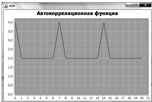
Рисунок 2 – Автокореляційна функція m -послідовності поліному 3го степеня
