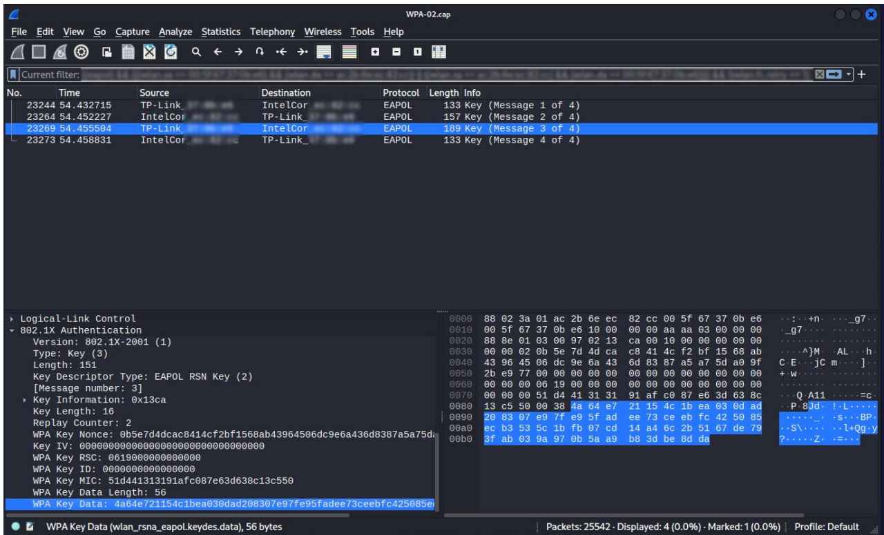
Рисунок 7.12 – Аналіз EAPOL пакетів у Wireshark
