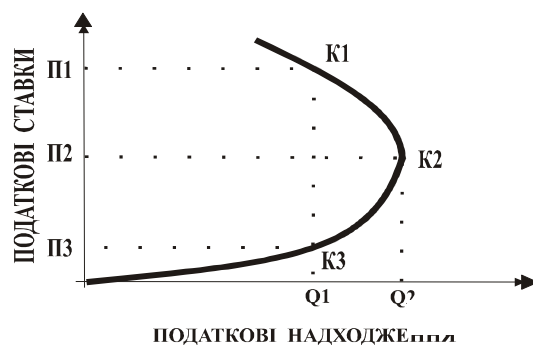
Рис. 1. Крива Лаффера
