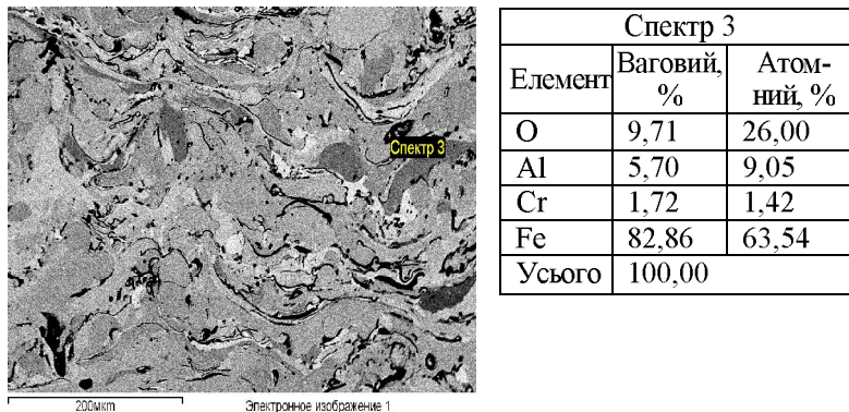
Рис.6. Структура та результати спектрального аналізу спектра 3 покриття 2 у відбитих електронах
