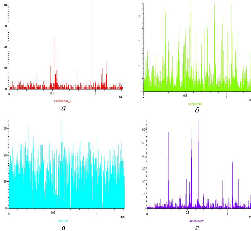
Рис. 8. Розподіл елементів у покритті з ПД 2: a – вуглець; б – оксиди; в – залізо; г – алюміній
