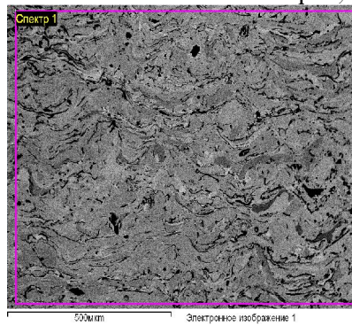
Рис. 5. Структура та результати спектрального аналізу спектра 1 покриття 2 у відбитих електронах
