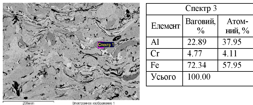
Рис. 7. Структура та результати спектрального аналізу спектру 1 покриття 2 у відбитих електронах
