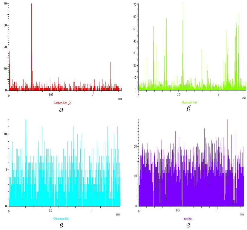
Рис.4. Розподіл елементів у покритті з ПД 1: a – вуглець; б – алюміній; в – хром; z – залізо
