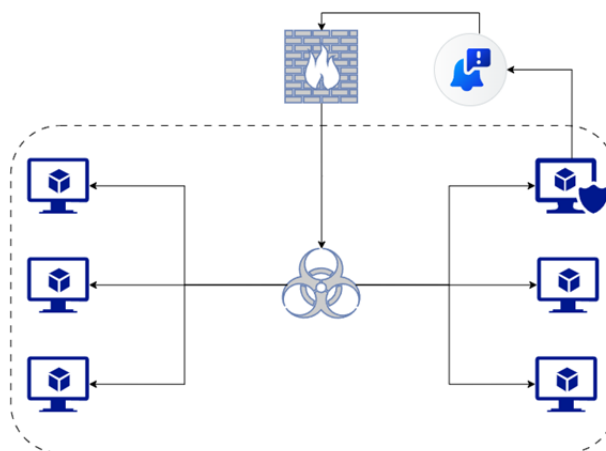
Рисунок 2 – Схема виявлення потенцїйних загроз за допомогою файлу honeypot
