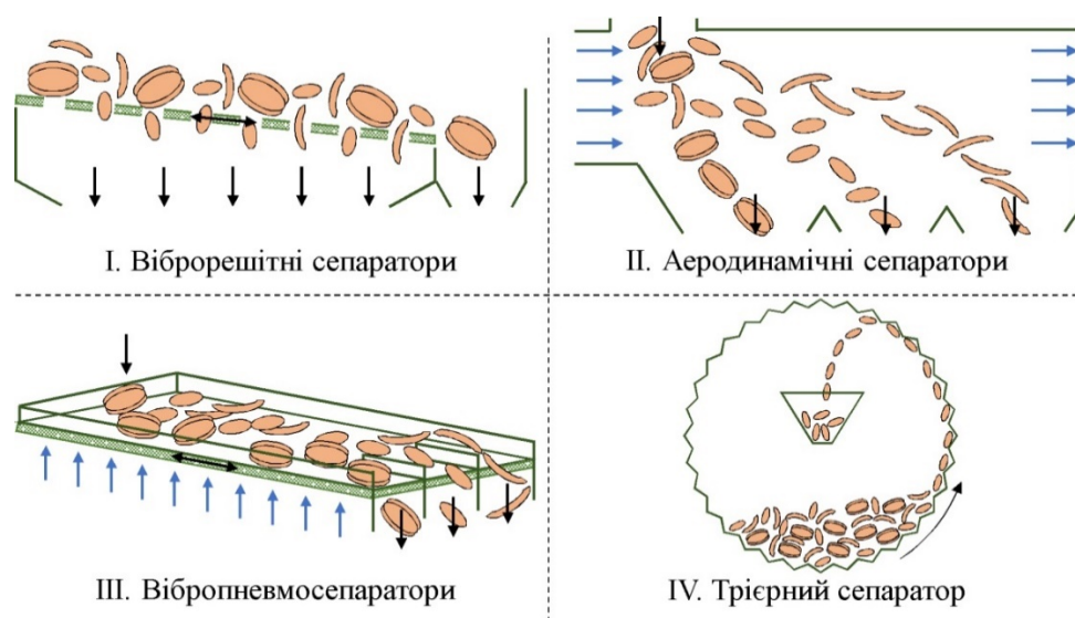
Рисунок 7 – Класифікація принципотих схем машин для очищення насінневої суміші
