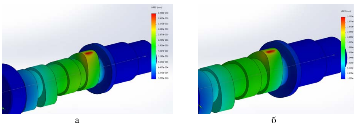
Рисунок 8 – Розподіл переміщення на поверхні кулачка розподільного вала: а – базовий варіант виконання розподільного валу; б – розподільний вал з кулачками, обробленими ФАБО
