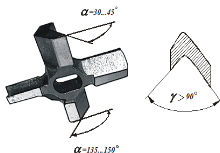
Рисунок 1 – Нож універсальний та перетин леза ножа універсального «розроблено авторами»
