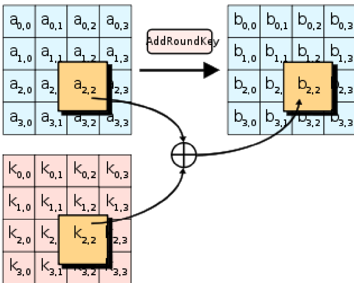
Рисунок 17.11 – Опис процедури AddRoundKey ()
