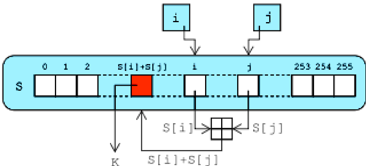
Рисунок 17.22 – Генератор ключового потоку RC4
