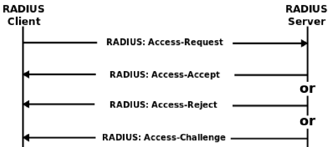
Рисунок 11.1 – Автентифікація та авторизація через RADIUS-сервер
