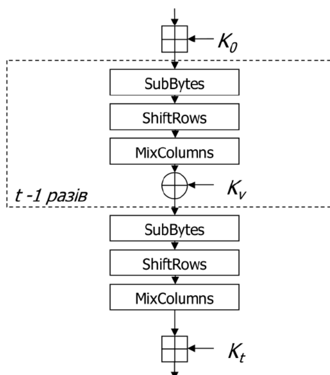
Рисунок 17.13 – Алгоритм шифрування «Калина»
