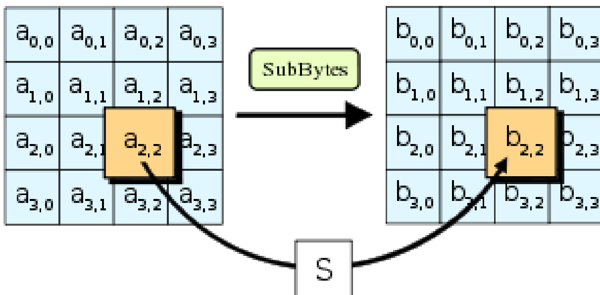
Рисунок 17.8 – Опис процедури SubBytes ()
