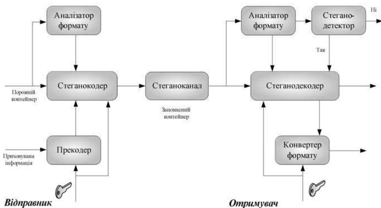
Рисунок 20.1 – Структурна схема типової стеганосистеми
