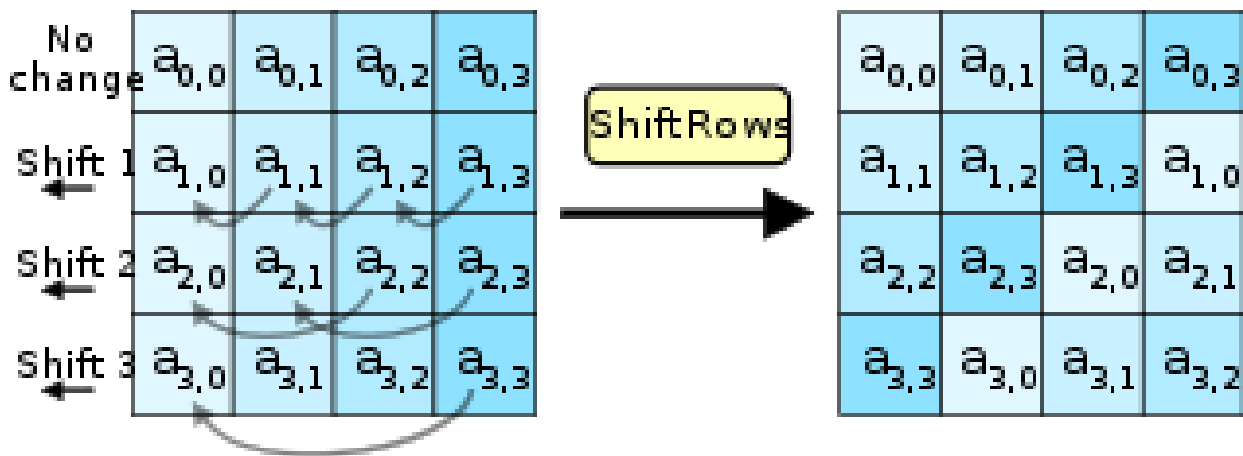
Рисунок 17.9 – Опис процедури ShiftRows ()
