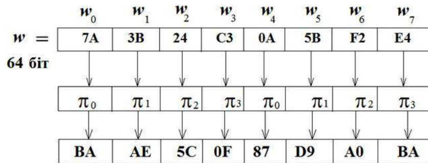
Рис. 17.25. Схематичне зображення виконання процедури підстановки T = T(w)
