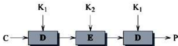
Рисунок 17.6 – Дешифрування потрійним DES
