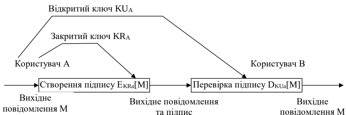
Рисунок 18.2 – Створення й перевірка підпису
