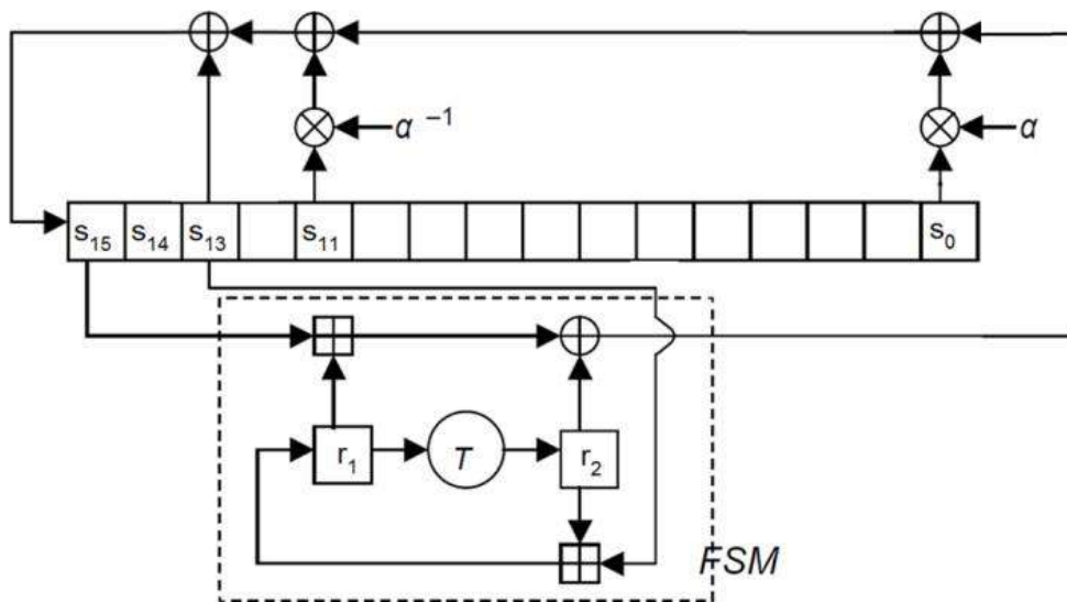
Рис. 17.24. Схематичне зображення генератору ключових потоків Струмок у режимі ініціалізації функції Next
