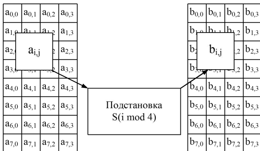
Рисунок 17.16 – Приклад підстановки байта для розміра блоку 256 біт
