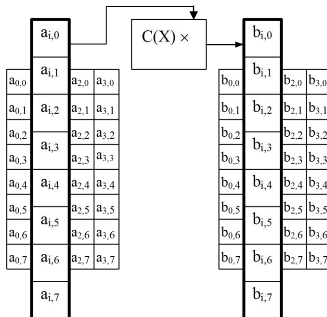
Рисунок 17.20 – Порядок виконання перетворення Mix Columns для поточного стану шифру з розміром блоку 256 біт
