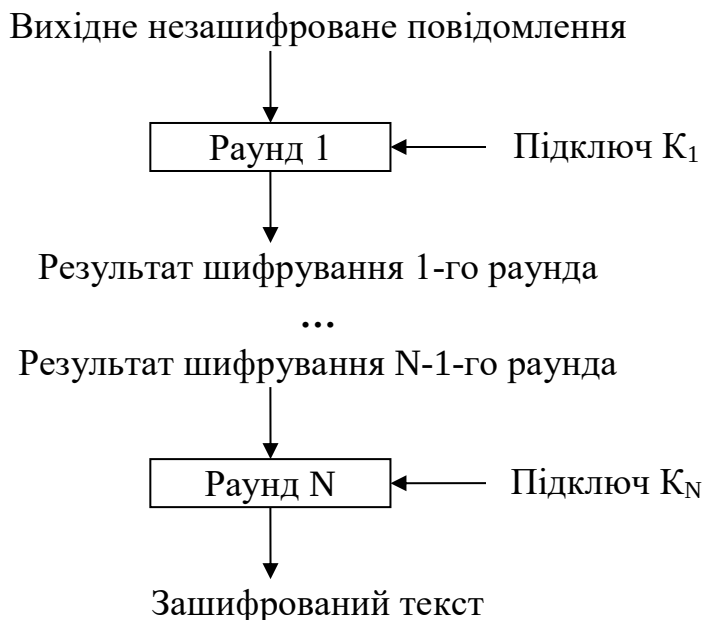
Рисунок 17.2 – Структура алгоритму симетричного шифрування
