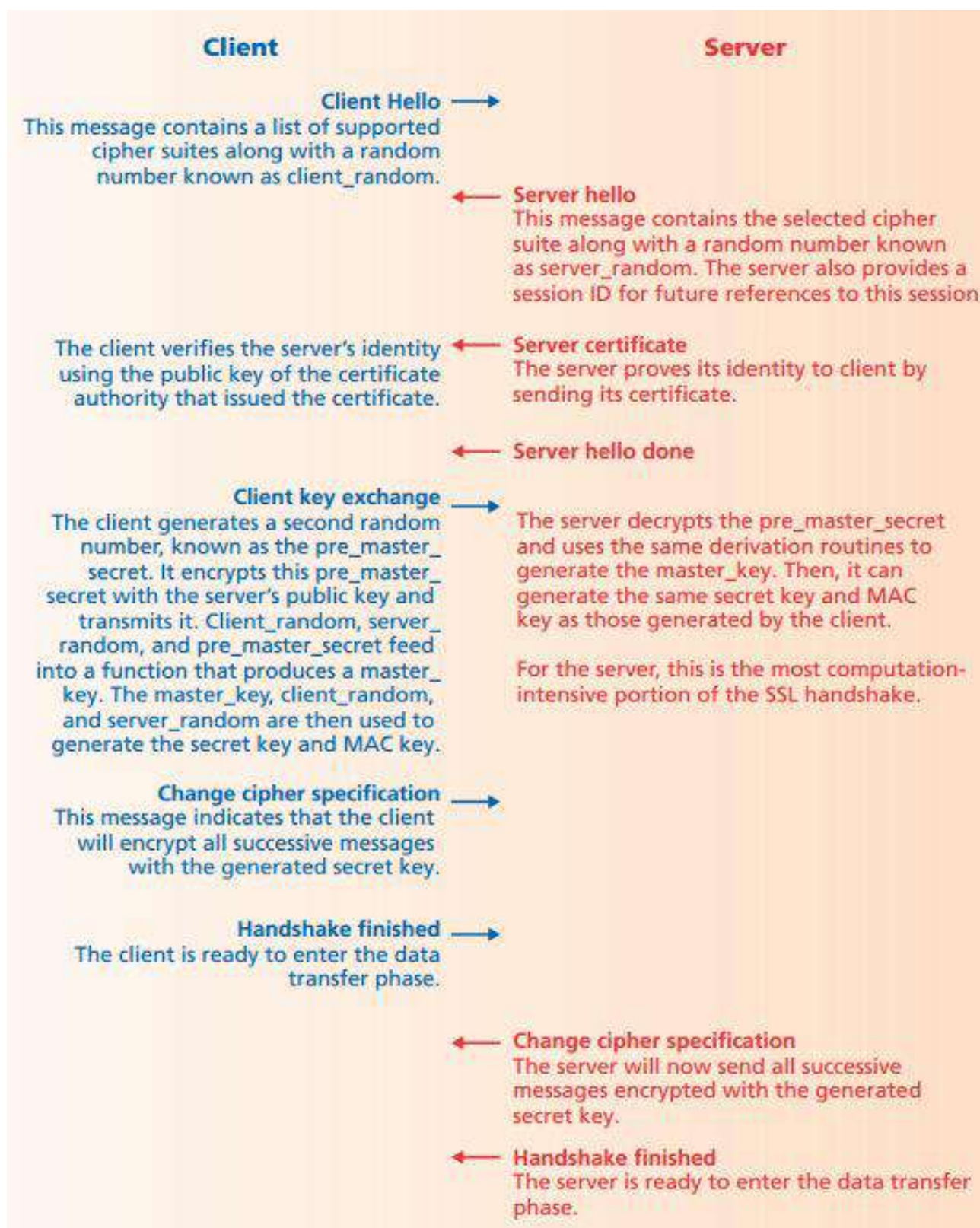
Рисунок 11.4 – Принцип роботи SSL
