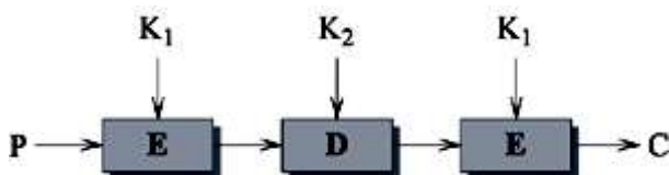
Рисунок 17.5 – Шифрування потрійним DES
