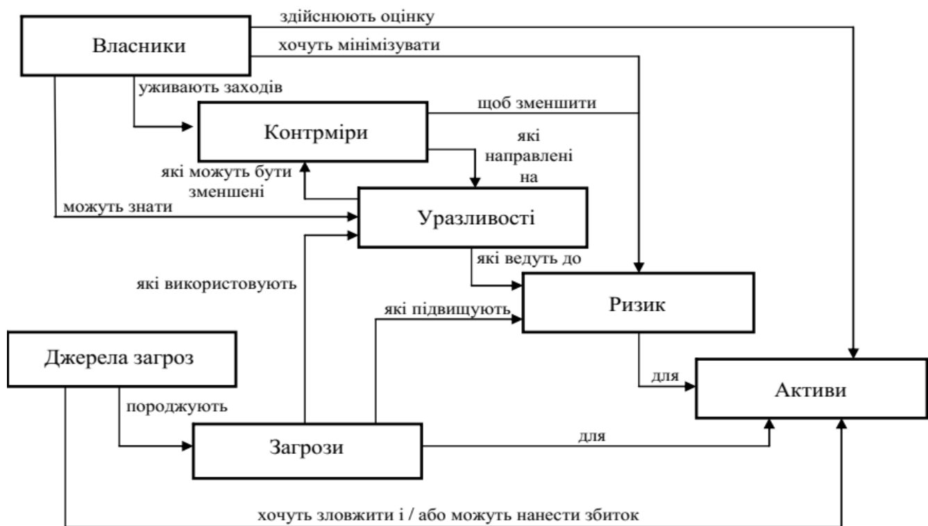
Рисунок 14.2 – Загальна схема забезпечення інформаційної безпеки відповідно до стандарту ISO/IEC 15408 «Критерії оцінки безпеки інформаційних технологій»
