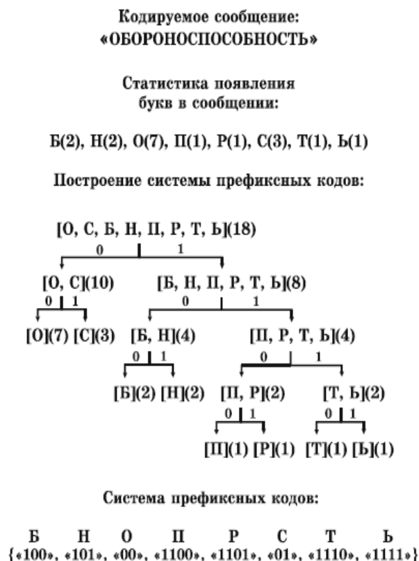
Рисунок 4.2 – Ілюстрація роботи алгоритму Шеннона-Фано на прикладі кириллиці
