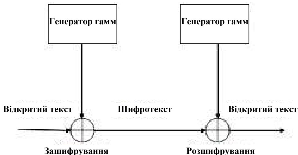
Рисунок 17.21 – Режим гамування для поточкових шифрів
