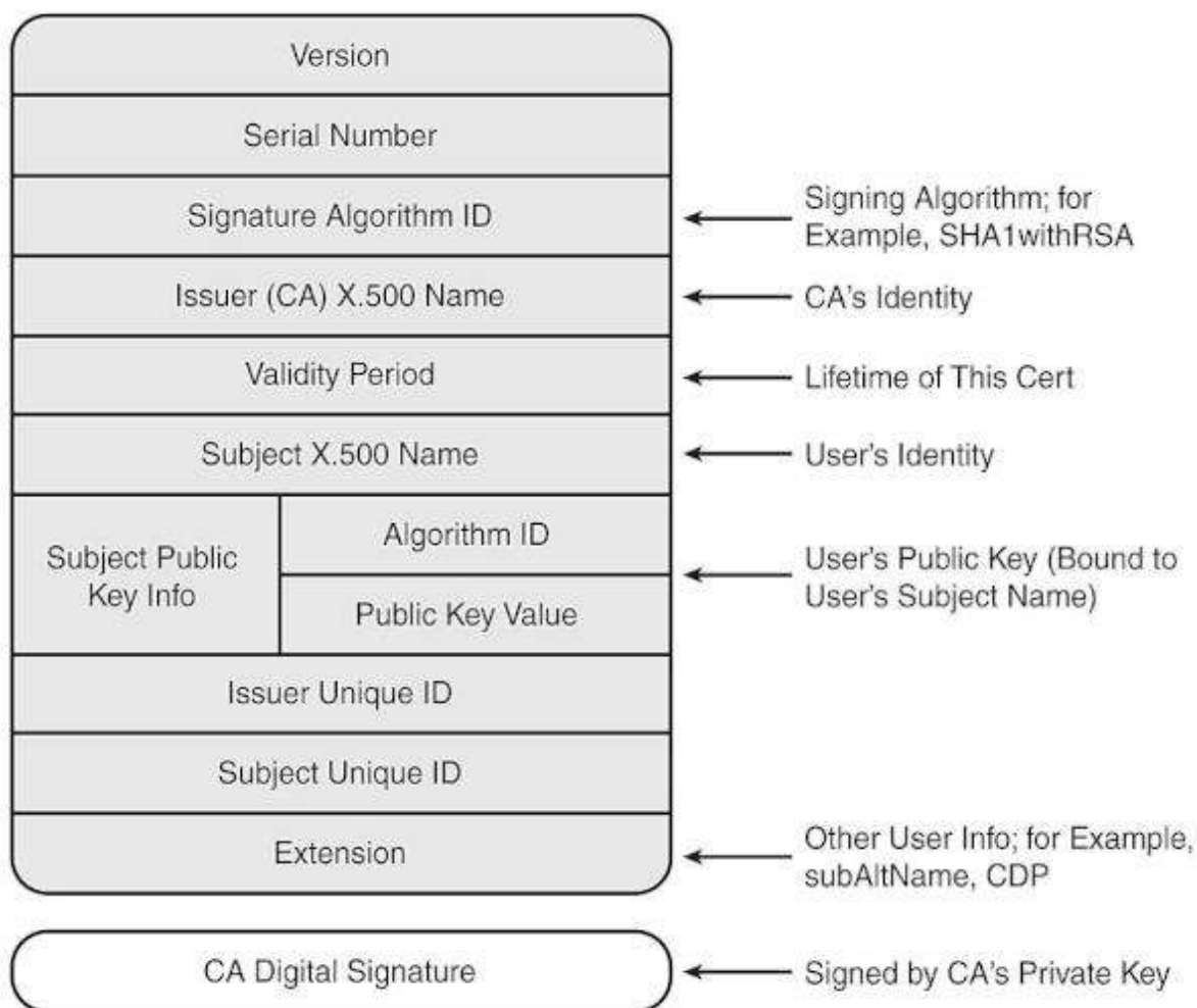
Рисунок 11.10 – Структура сертифікату X.509
