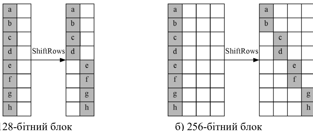
Рисунок 17.17 – Порядок розподілення байт першого стовбця при здійсненні перетворення ShiftRows
