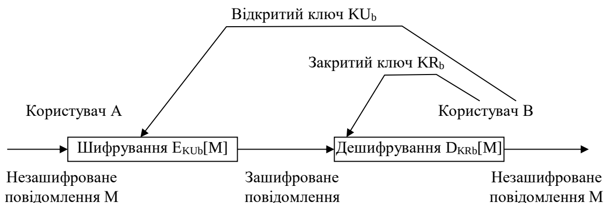
Рисунок 18.1 – Шифрування з відкритим ключем
