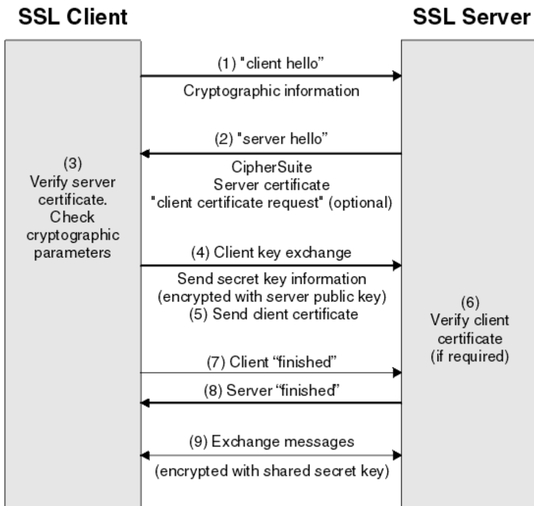
Рисунок 11.8 – Підтвердження зв'язку (handshake)
