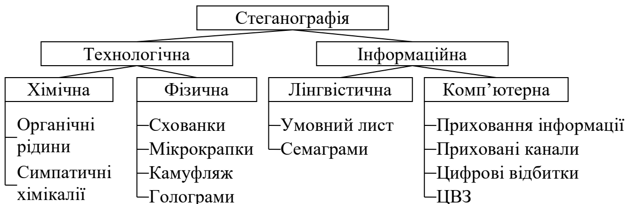
Рисунок 20.2 – Класифікація методів стеганографічного захисту
