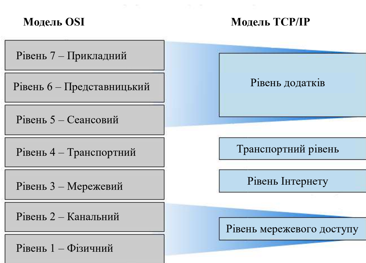
Рисунок 3.2 – Порівняння мережевих моделей OSI та TCP/IP
