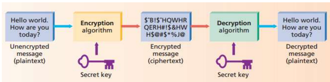
Рисунок 11.6 – Шифрування з використанням симетричних алгоритмів
