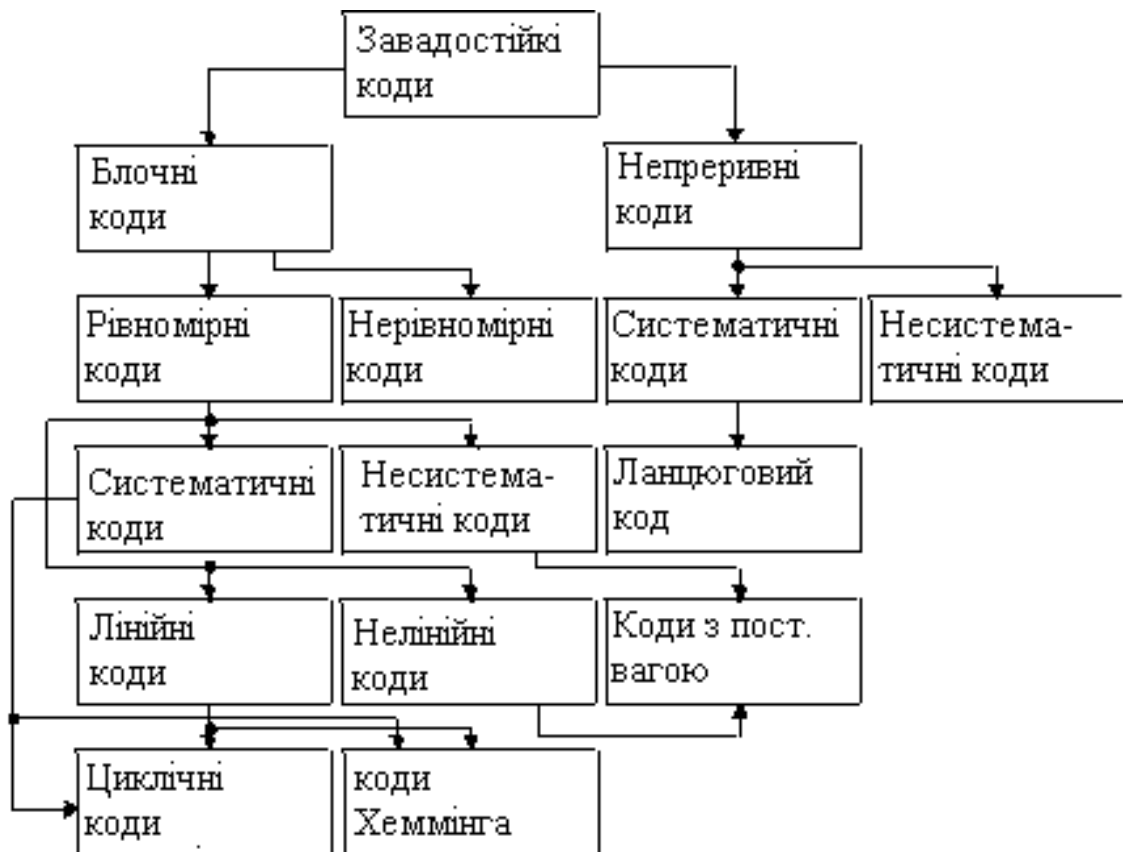
Рисунок 4.4 – Класифікація завадостійких кодів
