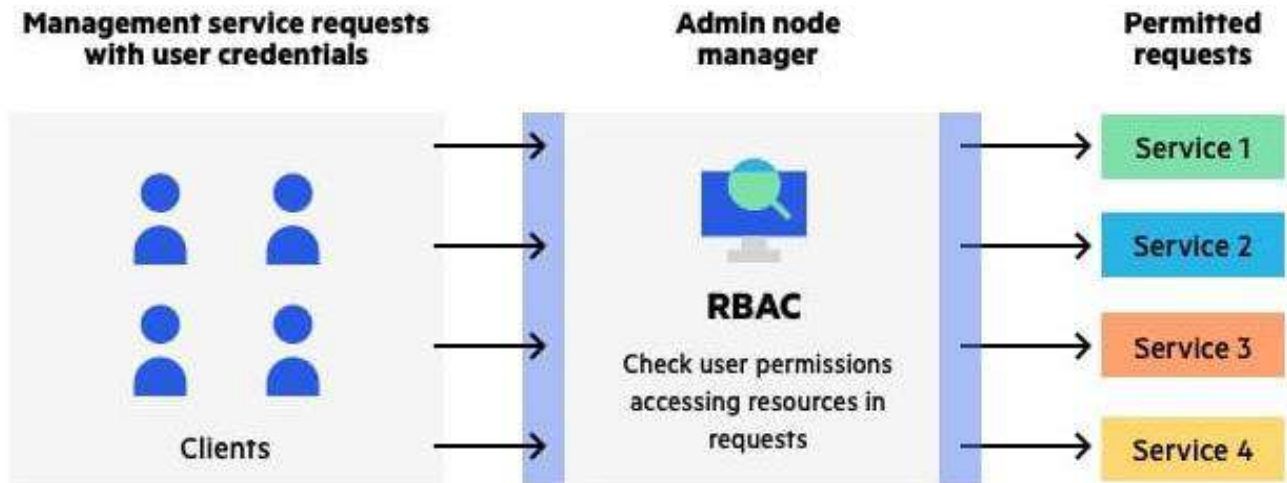
Рисунок 8.2 – Приклад системи керування доступом на основі ролей (RBAC)
