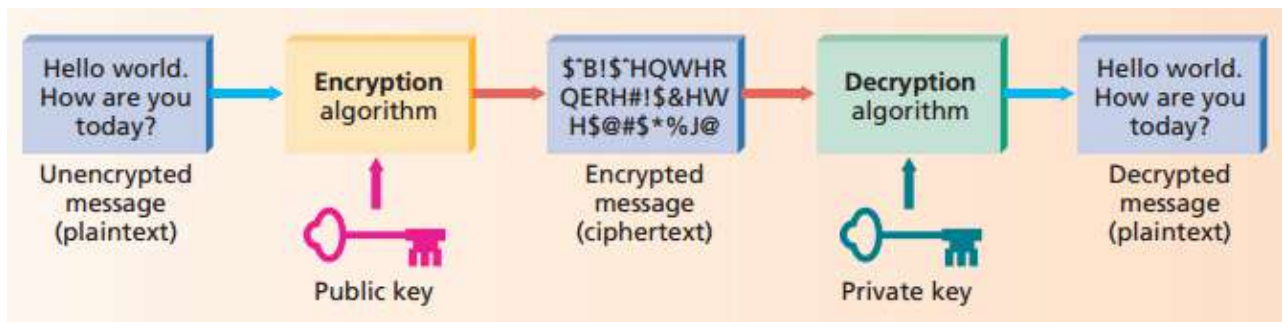
Рисунок 11.5 – Шифрування з використанням асиметричних (несиметричних, з відкритим ключем) алгоритмів
