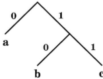
Рисунок 4.1 – Бінарне кодове дерево для системи префіксних кодів {«0», «10», «11»} (коди відповідають символам «a», «b» і «c»)
