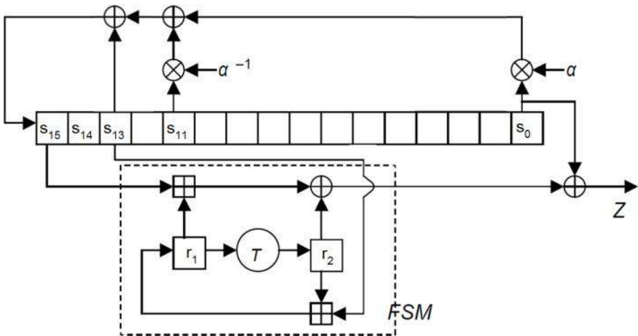
Рис. 17.23. Схематичне зображення генератору ключових потоків
