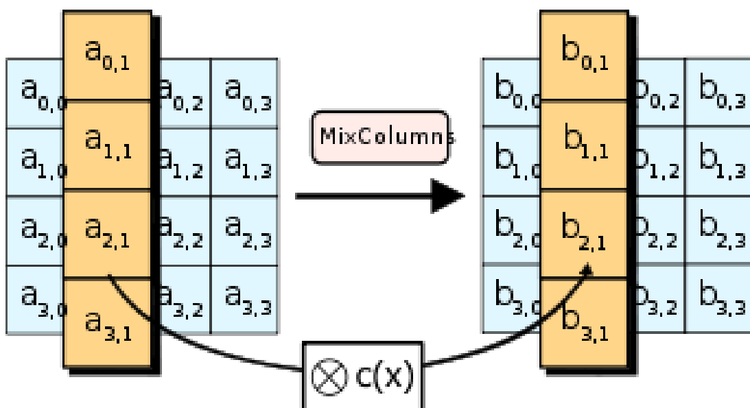
Рисунок 17.10 – Опис процедури MixColumns ()
