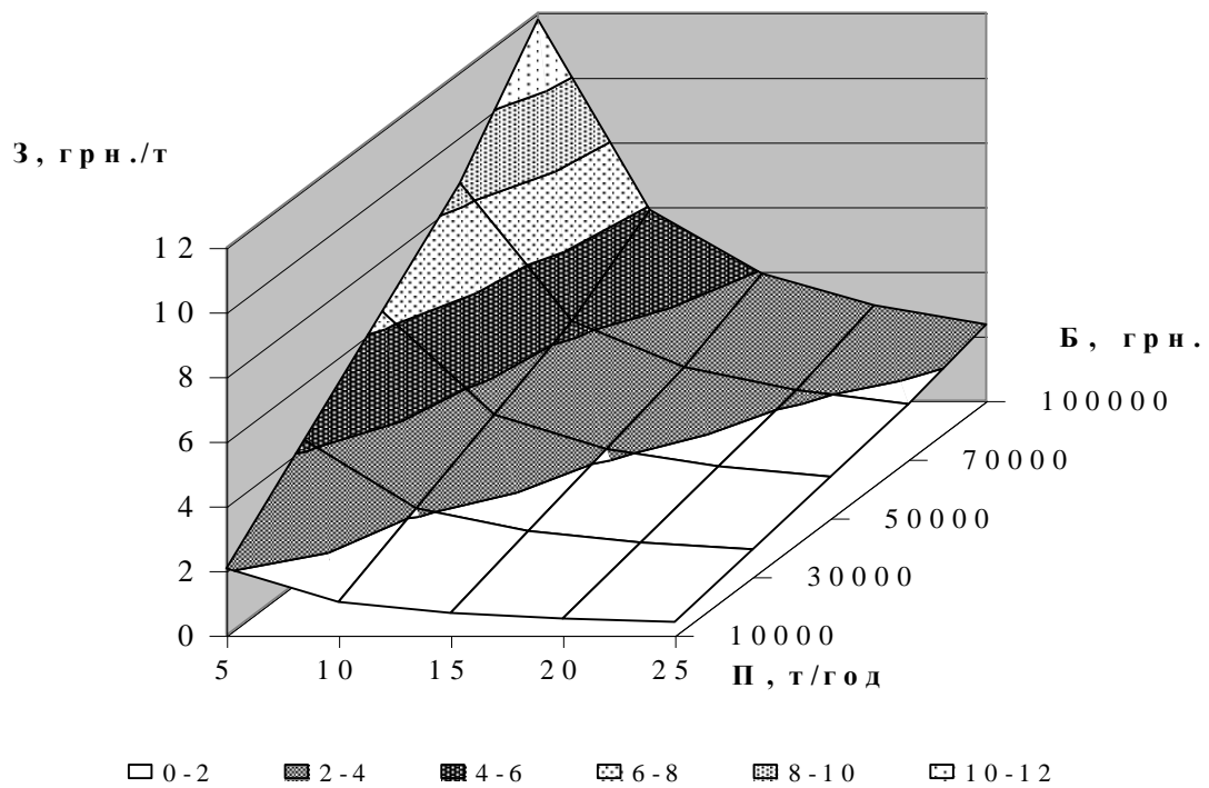
Рисунок 4 - Залежність питомих витрат на виконання технологічної операції сушаркою біогумусу від її продуктивності і балансової вартості
