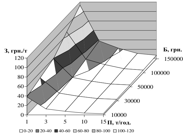
Рисунок 1 - Залежність питомих витрат на виконання технологічної операції відділювачем доштових черв'яків з субстратом від його продуктивності і балансової вартості
