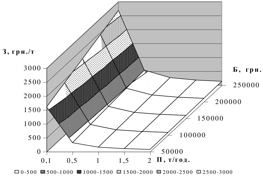
Рисунок 3 - Залежність питомих витрат на виконання технологічної операції відділювачем дощових черв'яків від вермикомпосту і сушіння біогумусу від його продуктивності і балансової вартості
