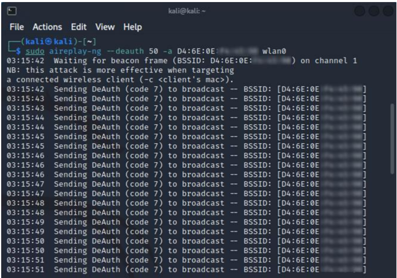
Рисунок 7.7 – Виконання ін’єкції команди для відключення від мережі
