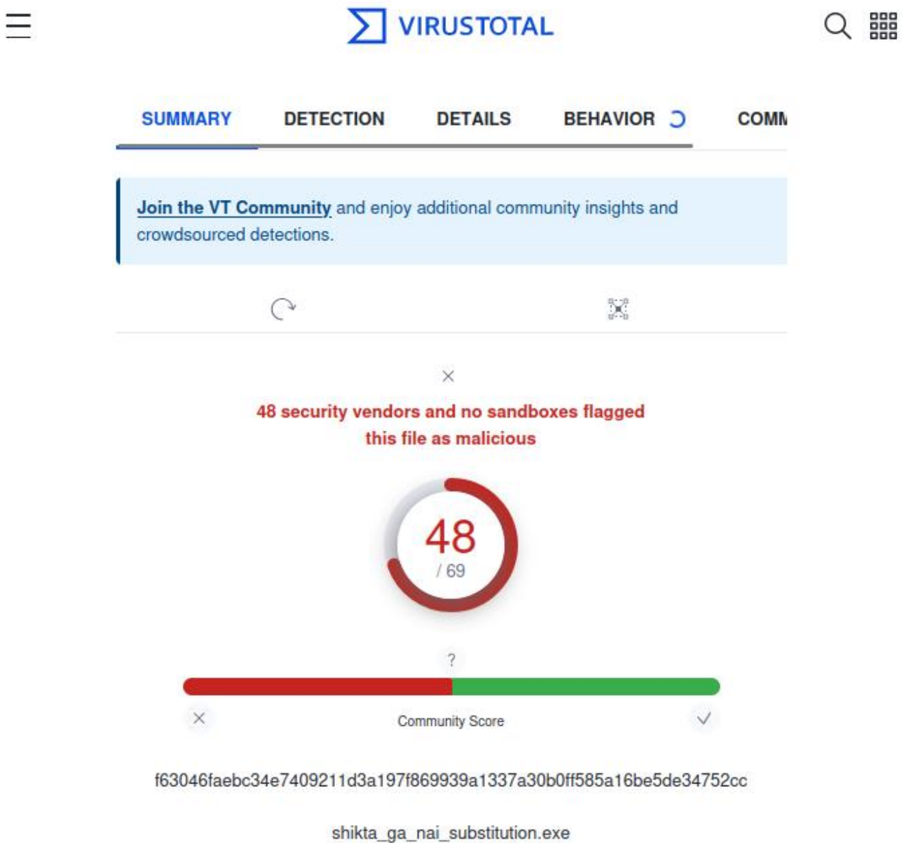
Рисунок 12.5 – Перевірка пейлоада за допомогою VirusTotal
