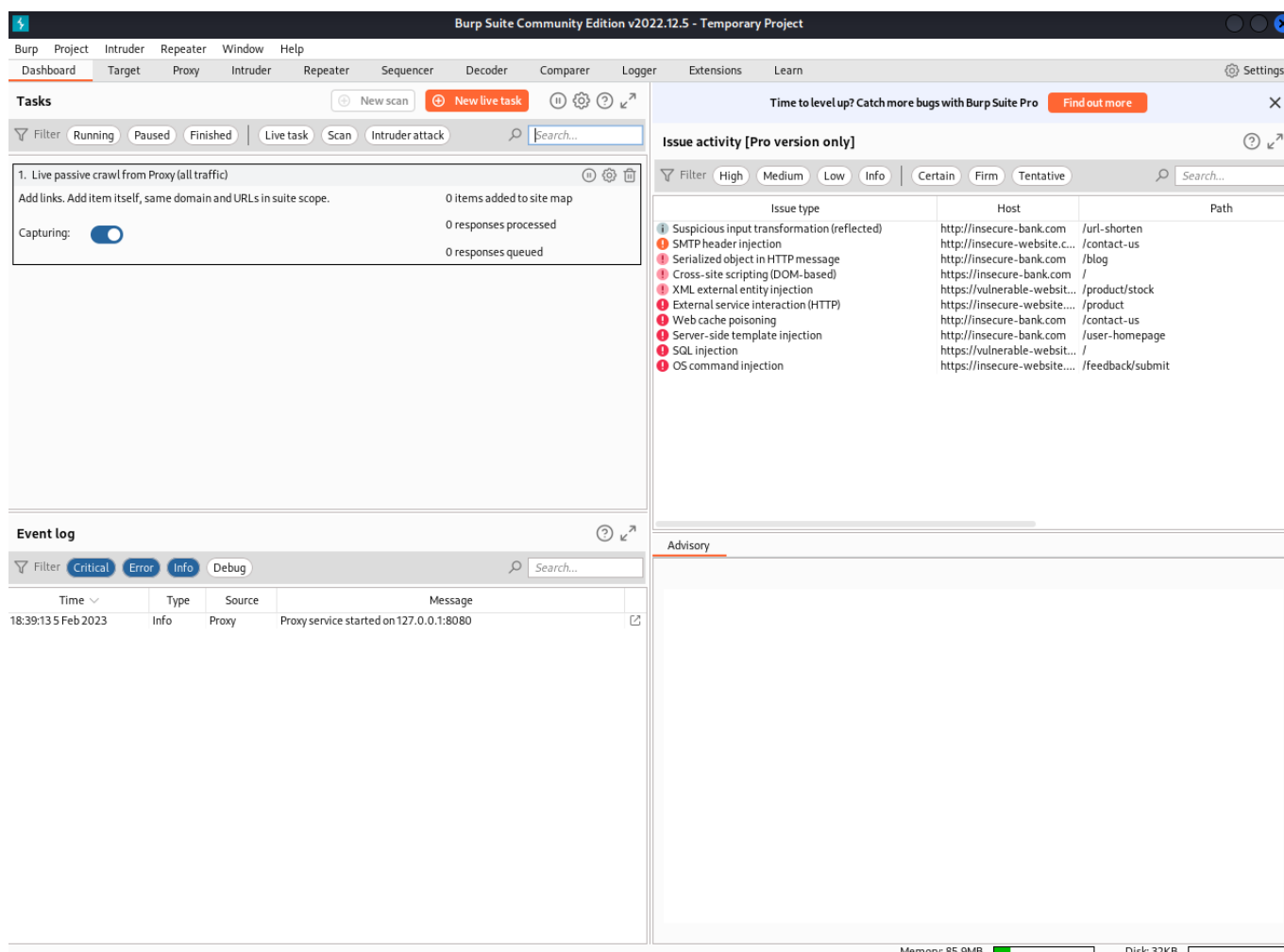
Рисунок 4.13 – Burp Suite
