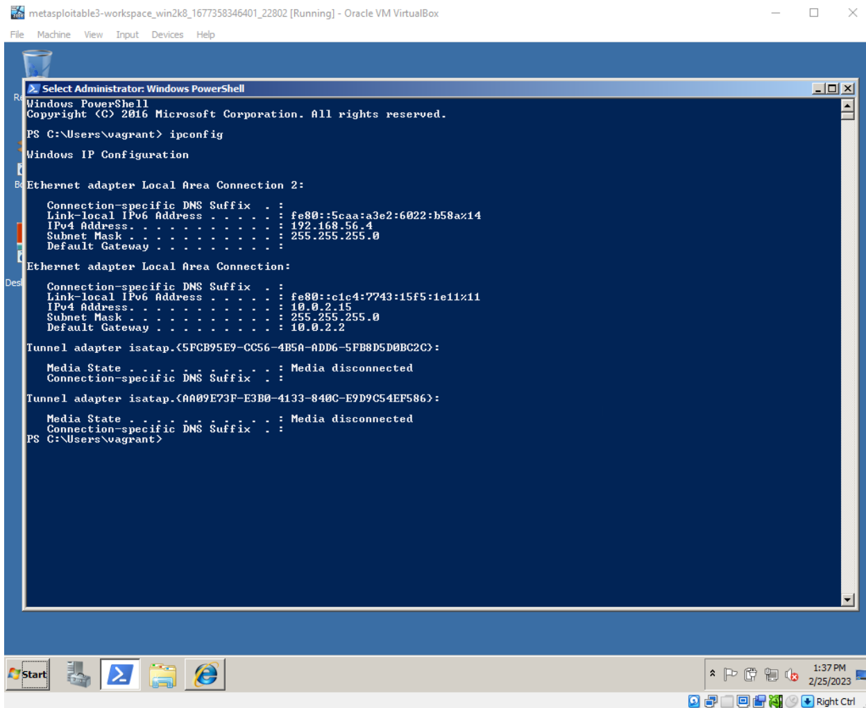
Рисунок 8.2 – IP-адреса Windows-машини
