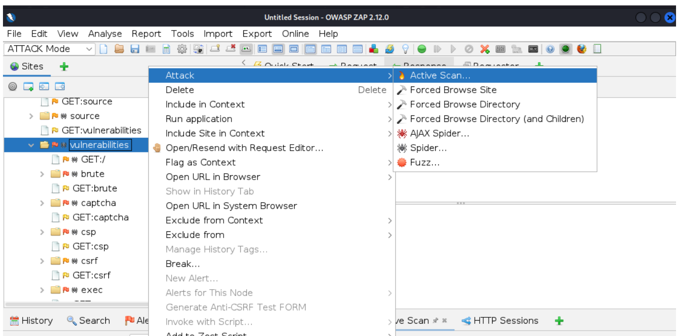
Рисунок 4.16 – Сканування окремої частини веб-додатка
