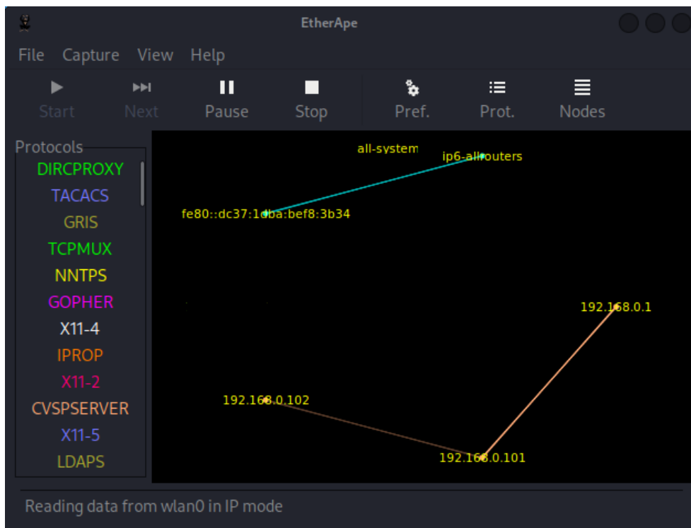
Рисунок 6.8 – Приклад роботи сніферу
