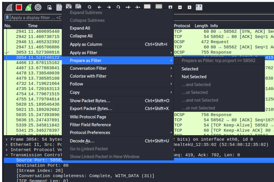
Рисунок 6.4 – Використання готового значення в якості фільтра
