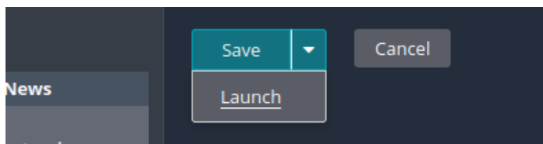
Рисунок 3.7 – Запуск сканування
