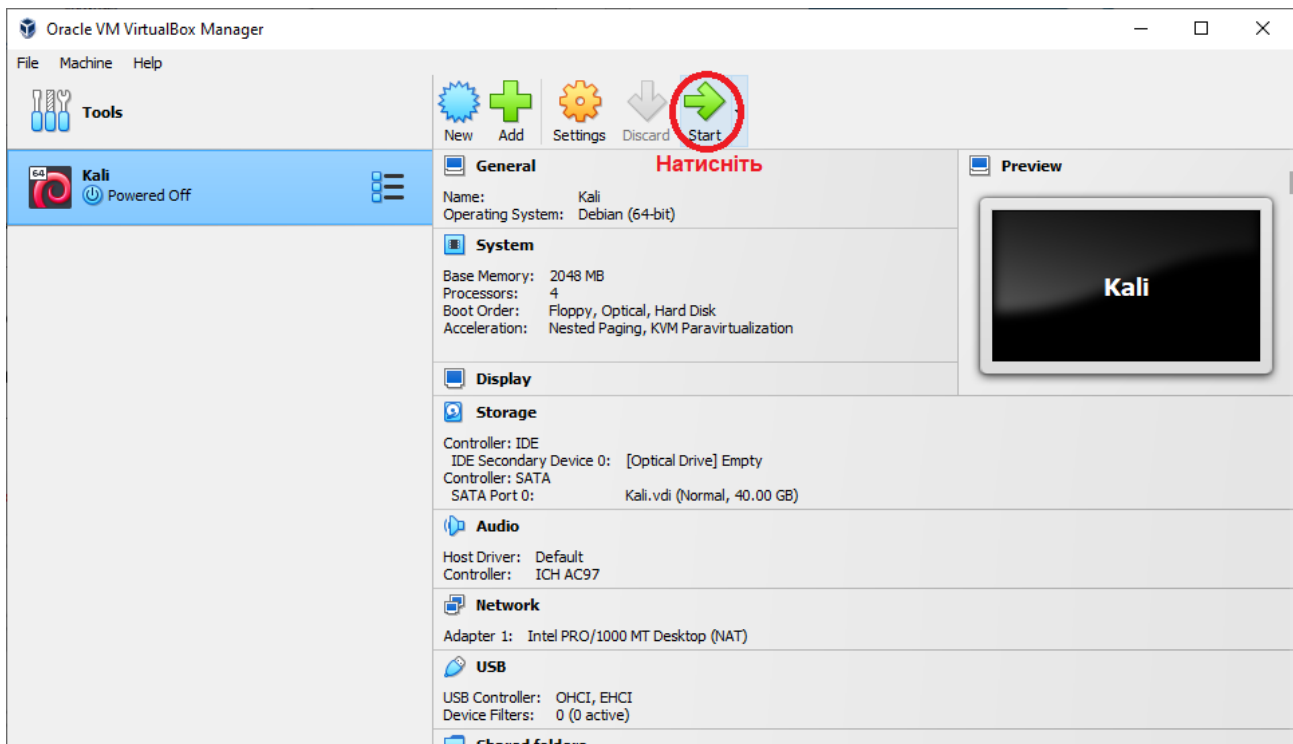
Рисунок 1.8 – Натисніть "Start"
