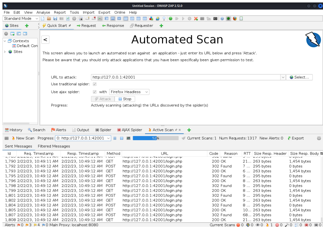
Рисунок 4.11 – Процес сканування
