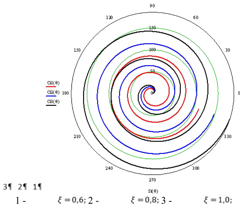
Рисунок 2 – Представлено геометрична інтерпретація моделі накладення шарів сипкого матеріалу над філь'єрою матриці на торцеву поверхню гранули для різних значень параметра \xi Джерело: розроблено авторами
