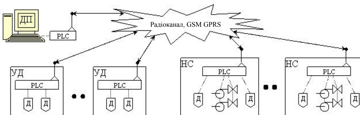
УД - удалений датчик; НС – насосна станція; ДП – диспетчерський пункт Рисунок 1 – Узагальнена структура АСУ
