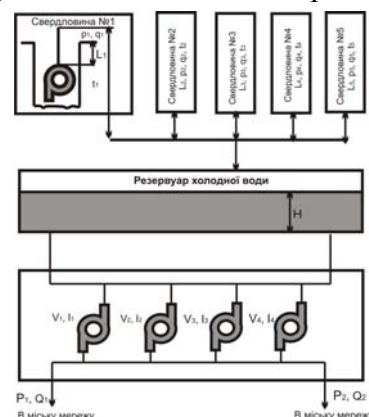
Н-рівень води в резервуарі; I-струм насосу станції; P-тиск на виході станції; Q-витрата води на виході станції; V-швидкість обертання валу двигуна насосу; L-рівень води в свердловині; r-тиск води в свердловині; q-витрата води в свердловині; t-температура повітря Рисунок 3 – Структурна схема Кіровоградського водоканалу
