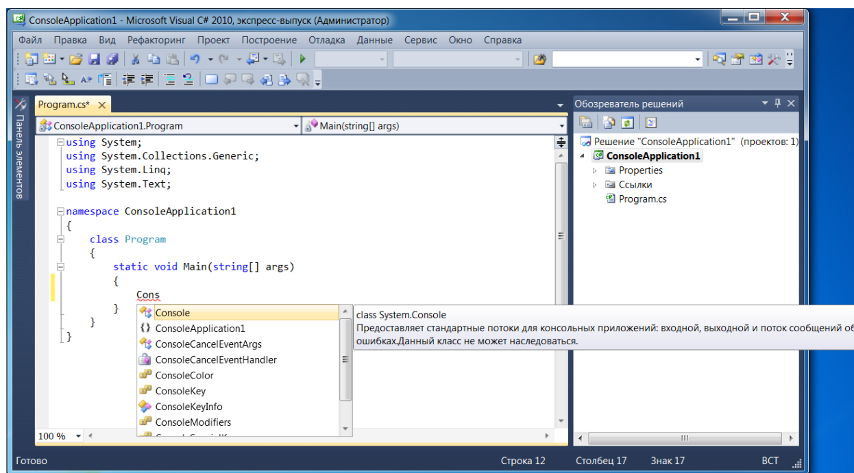
Рисунок 1.5 – Використання IntelliSense
