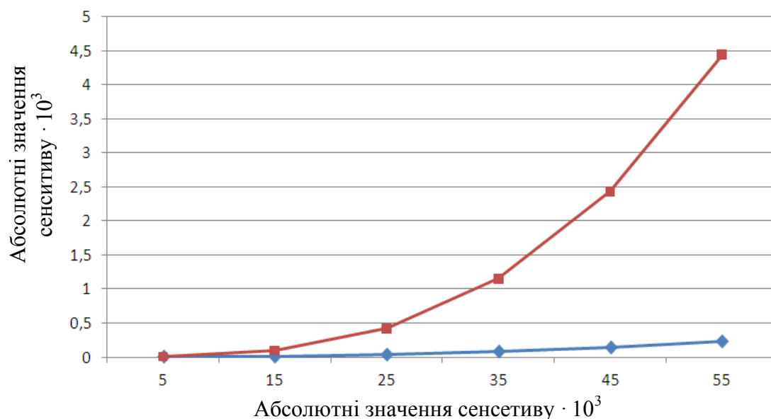
Рис.2 – Залежність чутливості діагностичного параметру агрегату від пробігу автомобіля: — ромб — чутливість температури спалаху оливи, — квадрат — чутливість діелектричної проникності оливи.
