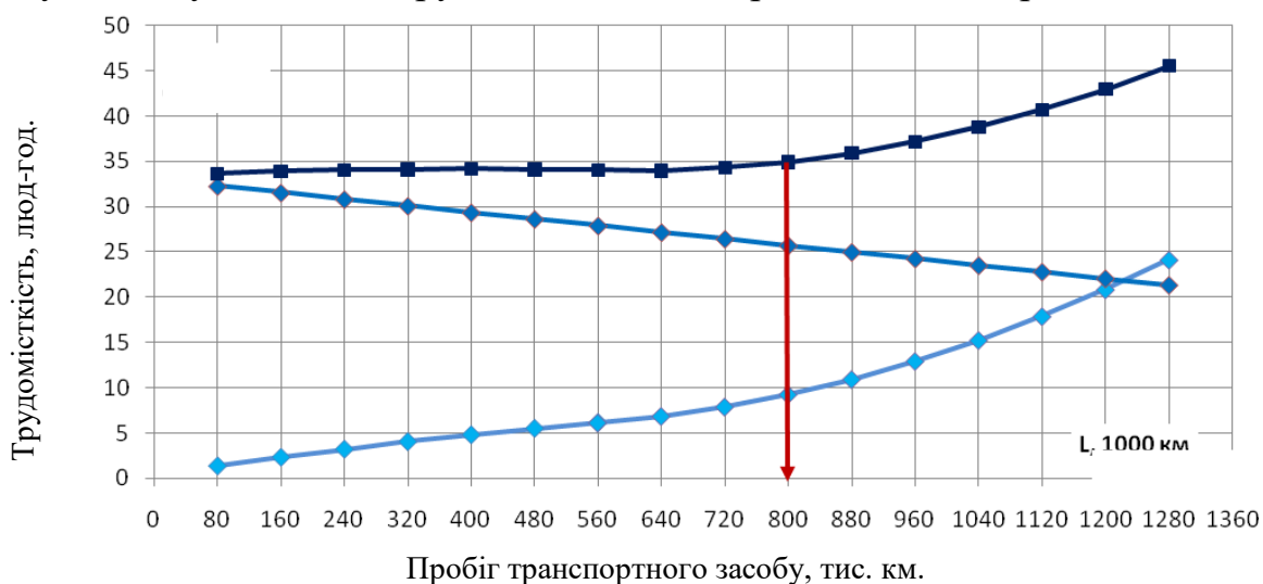
Рисунок 10 – Визначення величини пробігу ефективної експлуатації сідельних тягачів "Scania": — ромб світло-синій - трудомісткість ПР; — ромб темно-синій - трудомісткість ТО; — квадрат темно-синій - сума ТО і ПР
