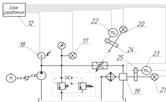
Рисунок 2 – Система автоматизованого керування гідравлічним пристроєм: 12 – блок управління; 17 – датчик тиску; 18 – датчик температури; 19 – термодатчик; 20, 21 – датчики положення; 22, 23 – крокові двигуни; 24, 25 – редуктора
