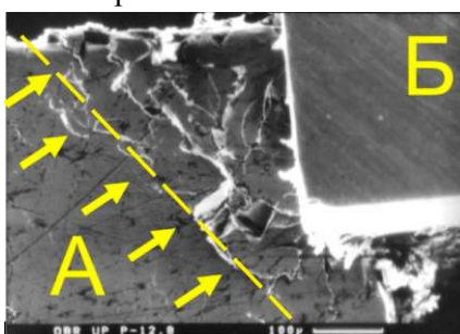
Рис. 8. Розвиток зони стружкоутворення: А - зразок, Б - ріжучий елемент
