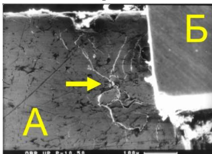
Рис. 7. Виникнення зони стружкоутворення: А - зразок, Б - ріжучий елемент
