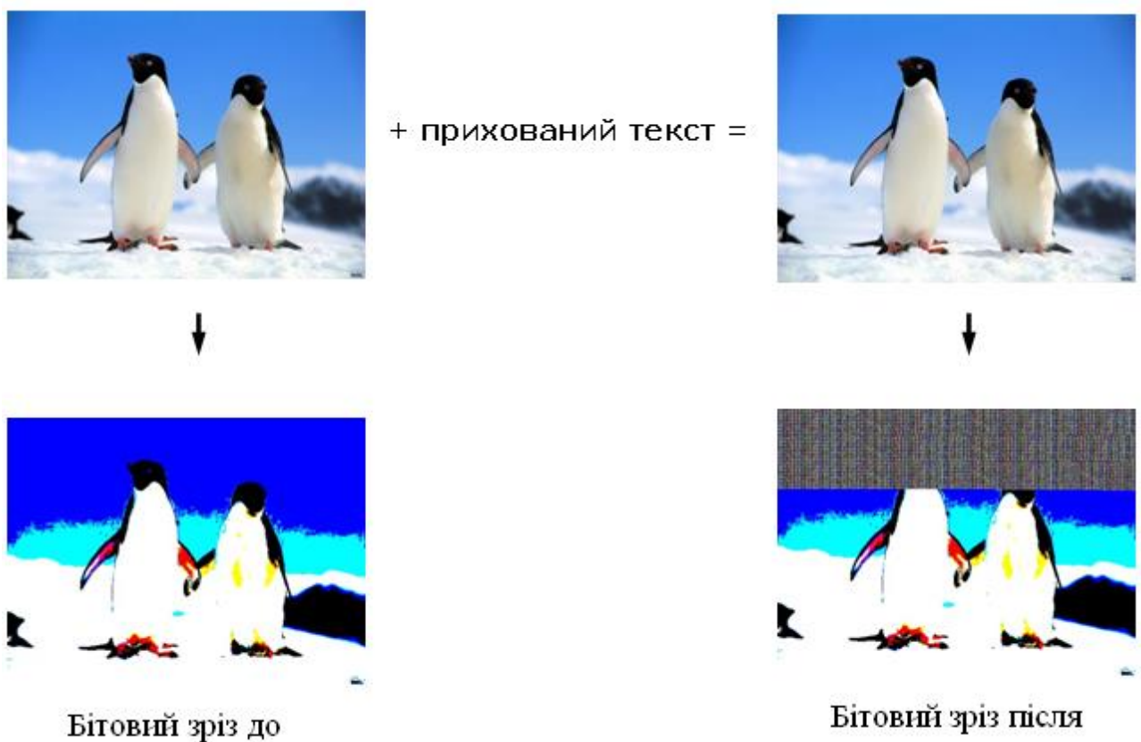
Рисунок 1 – Вигляд бітового зрізу файлу до та після вдубовування текстового повідомлення методом LSB
