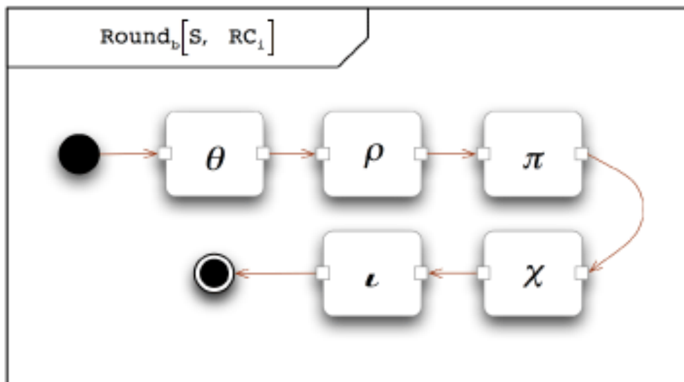
Рисунок 6 – Цикл перетворення SHA-3 (Кессак)
