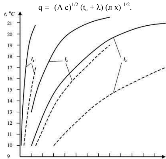
Рис.4. Залежність зміни температури підзолистого ґрунту від часу при різних відстанях від зовнішньої стінки ТЕ акумулятора I ( l_1 = 0,1 м; l_2 = 0,2 м; l_3 = 0,3 м) та різних w , %: штрихова — 10; суцільна — 25.
