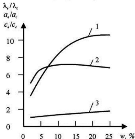
Рис.1. Залежність відношень коефіцієнтів теплопровідності, температуропровідності та теплоємності від вологості для супіску: 1 - ХвАс; 2 - аλ/аλ, 3 - Св/Сс.
