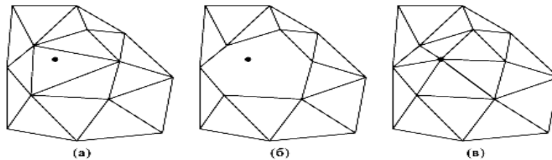
Рисунок 1 – Приклад алгоритму «Видаляй та будуй»
