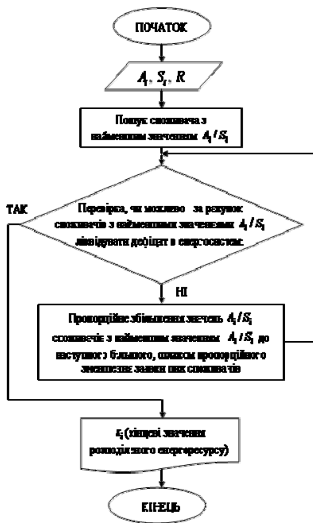
Рисунок 1 – Схема розрахунку методом ітераційного розподілу енергоресурсу
