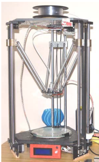
Рисунок 4 – 3D-принтер DELTA-FDM
