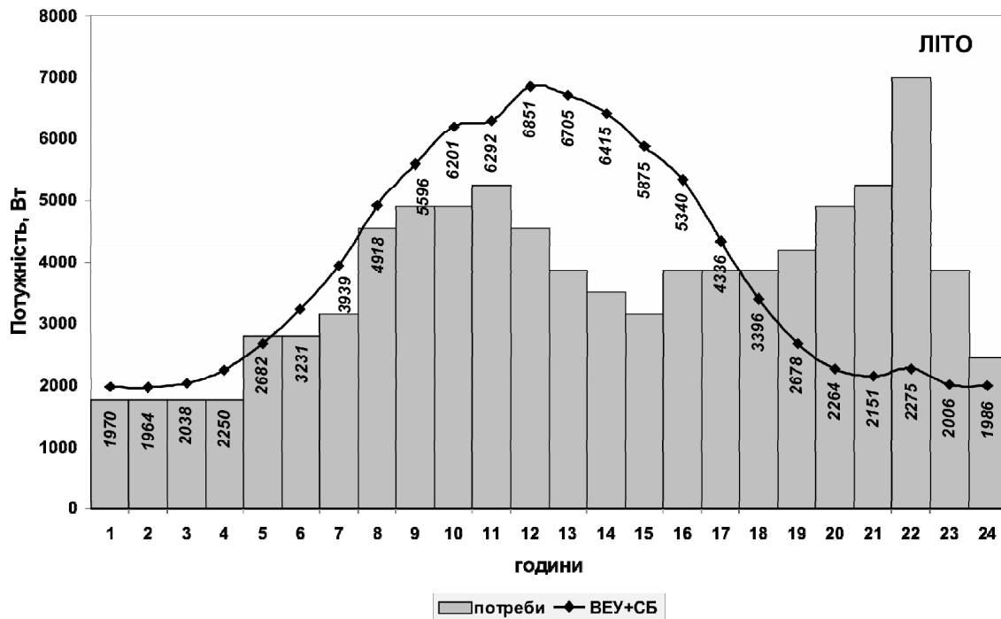
Рисунок 6 – Середньодобовий графік енергетичних потреб фермерського господарства та сумарної кількості енергії літню
