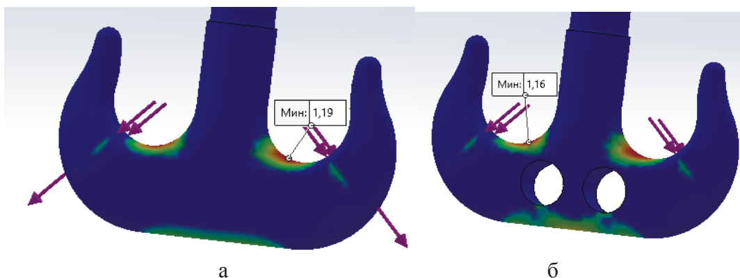
Рисунок 10 – Розподілення напружень в елементах моделі при схемі навантаження №1 (рис. 4)
