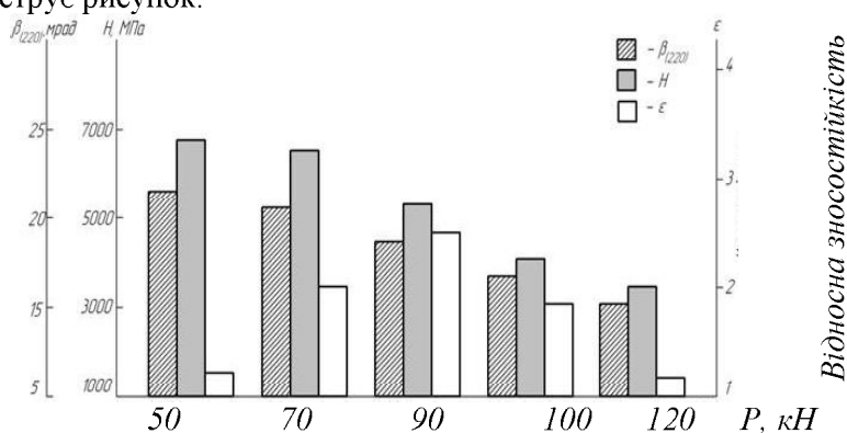
Вплив зусилля деформації P на мікротвердість H , фізичне розширення рентгенівських ліній \alpha -фази \beta_{(220)} і відносну зносостійкість \epsilon сталі 40X
