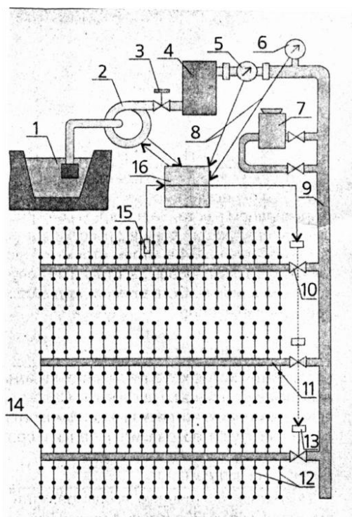
Рис. 6.1. Принципова схема системи крапельного зрошення:
