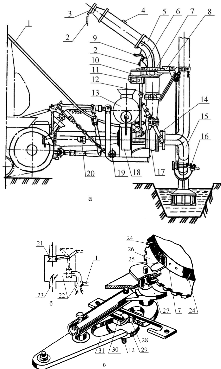
Рис. 21. Далекоструминний начіпний дощувач
