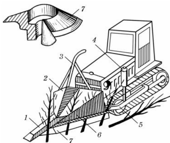
Рис. 1.1. Кущоріз ДП-24
