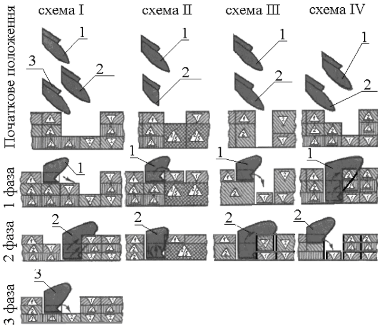
Рис. 3. Технологічний процес роботи при триярусній оранці
