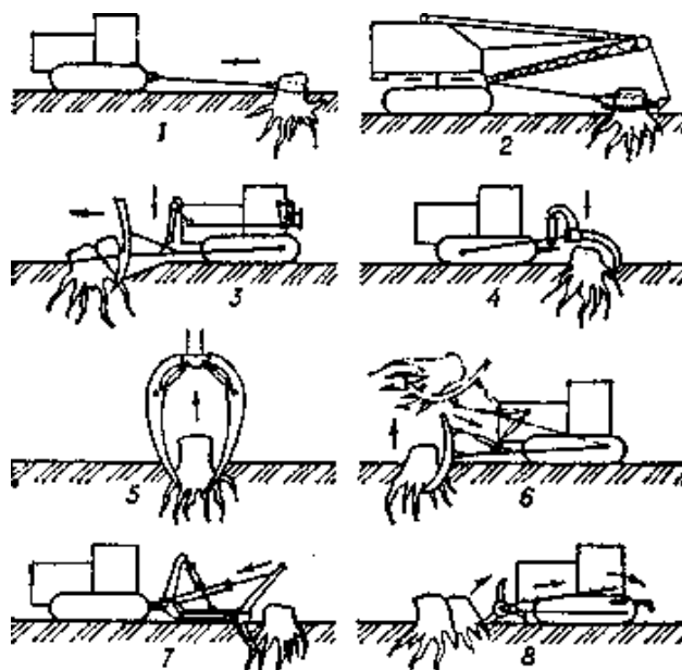
Рис.1.2. Схеми корчувальних машин :
