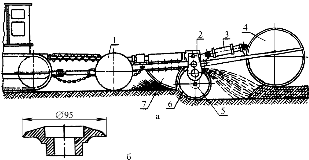
Рис. 8. Машина для глибокого фрезерування МТП-42
