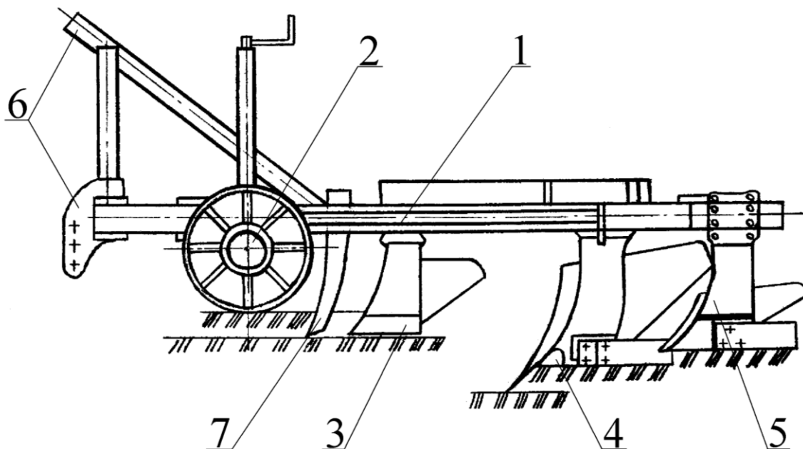
Рис. 2. Загальний вид плуга ПТН-40
