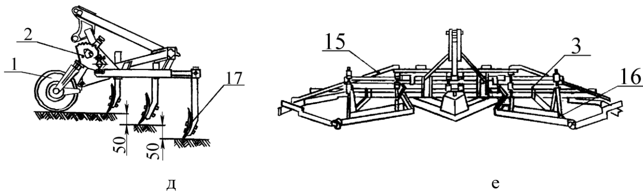
Рис. 10. Універсальний каналокочач–зарівнювач КЗУ–0,3
