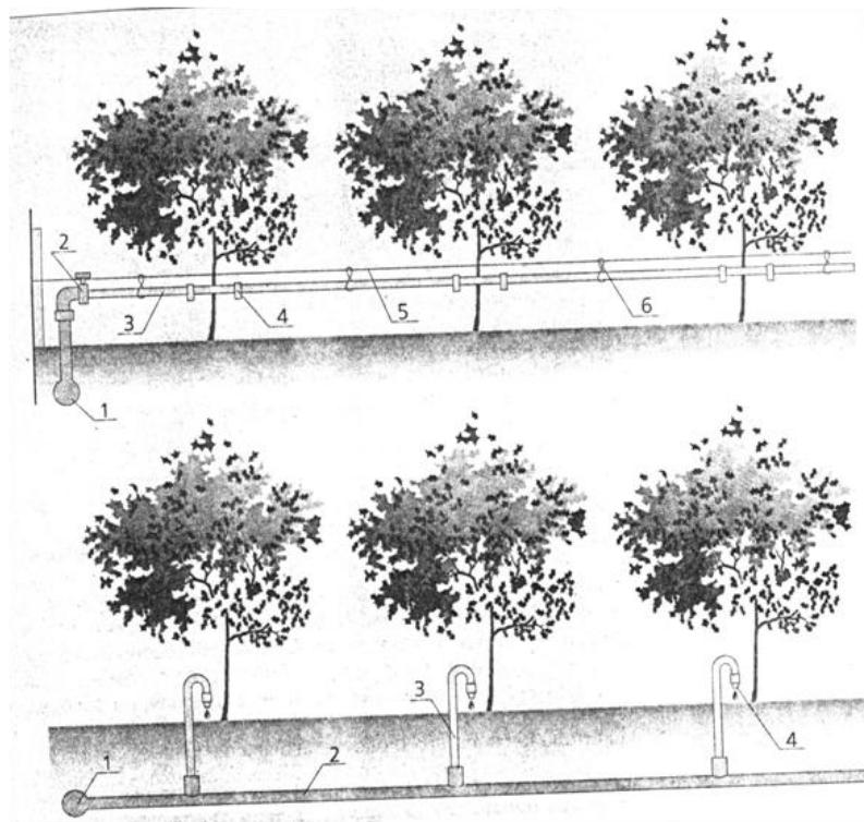
Рис.6.2. Схеми розміщення поливних трубопроводів системи крапельного зрошення:
