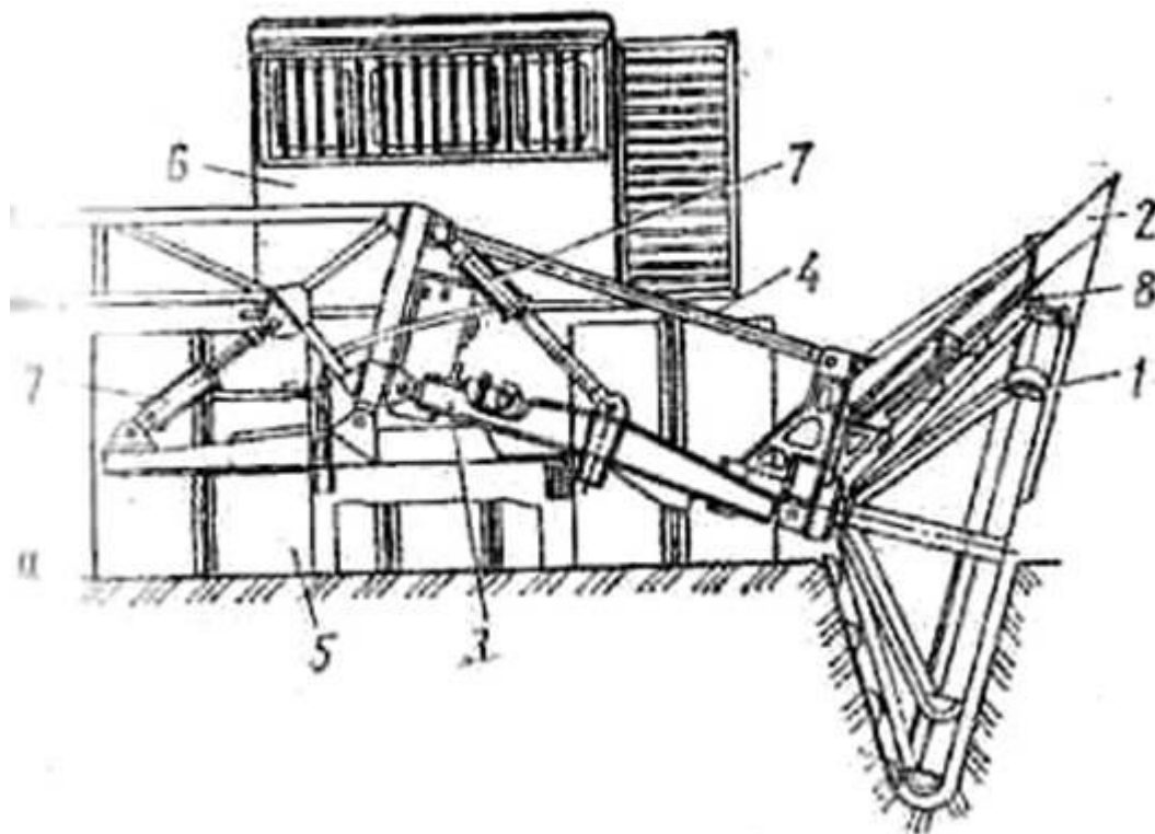
Рис. 7.4. Причіпний фрезерний каналокпач з копіювальною фрезою: 1 – фреза; 2 – напрямний козирок; 3 – виносна рама (стріла); 4 – верхній важіль навіски; 5 – опорні котки; 6 – трактор; 7 – гідроциліндр; 8 – чашковий ніж.
