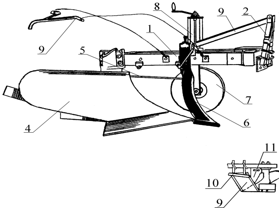
Рис. 4. Загальна будова чагарниково–болотного плуга ПБН–75
