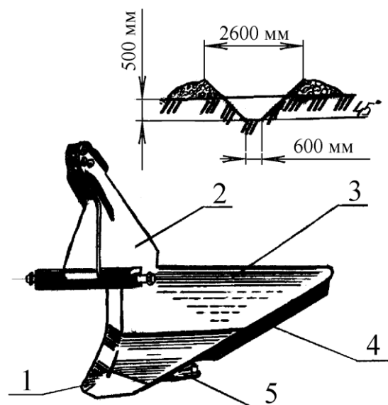
Рис. 11. Каналокопач Д-716
