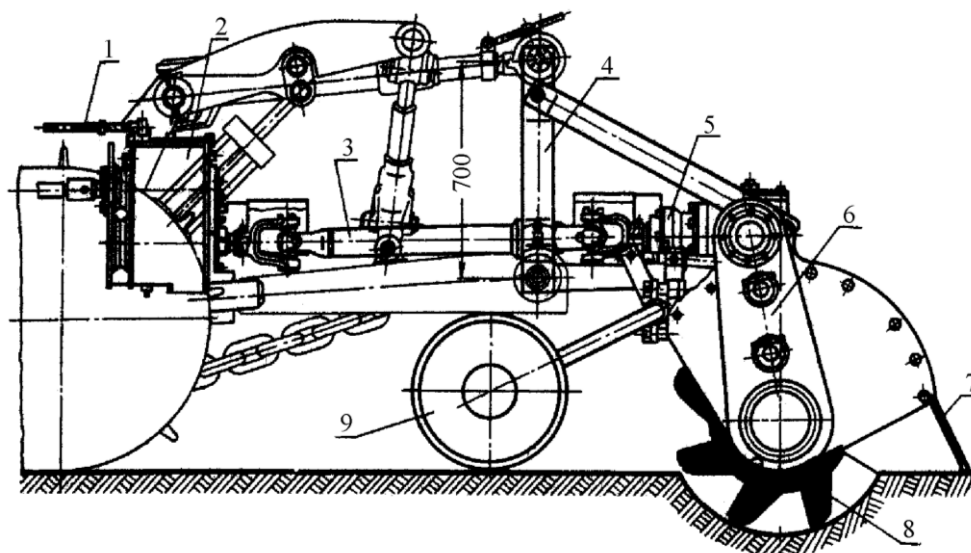
Рис. 7. Болотна фреза ФБН-2,0
