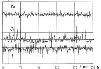
Рисунок 5 – Осцилограми РОД калібрування припуску 2-4 мм: а – 25В, 70А, 0,6МПа; б – 32В, 100А, 0,5МПа; в – 25В, 150А, 0,8МПа
