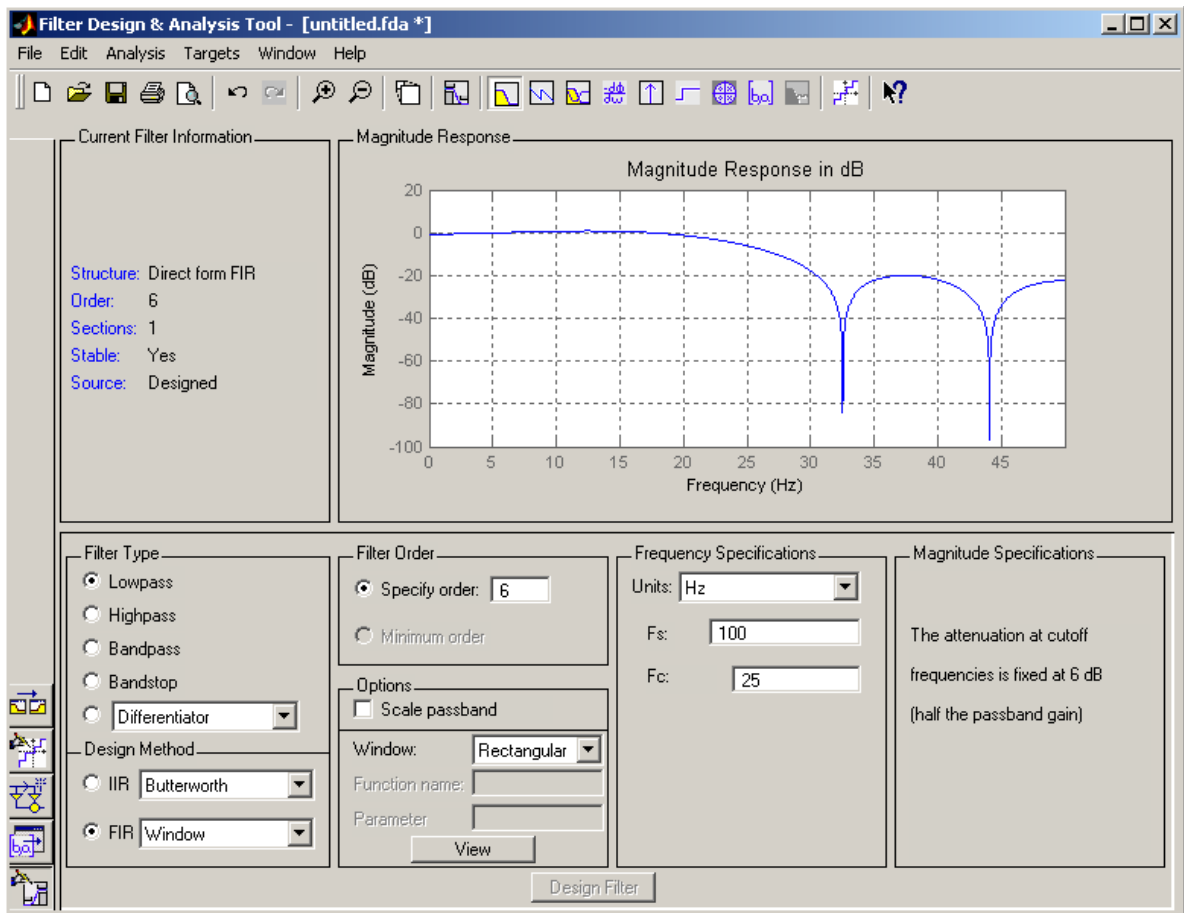
Рис.2.13. Вікно fdatool
