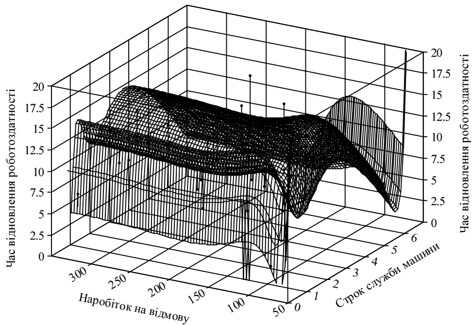
Рисунок 1 – Графік залежності часу на відновлення роботоздатності від наробітку на відмову та строку служби кормодробарок
