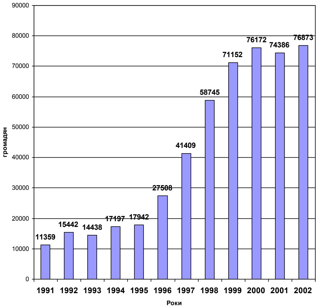
Рисунок 3 – Чисельність незайнятих громадян, які перебували на обліку в службі зайнятості у 1991-2002 рр
