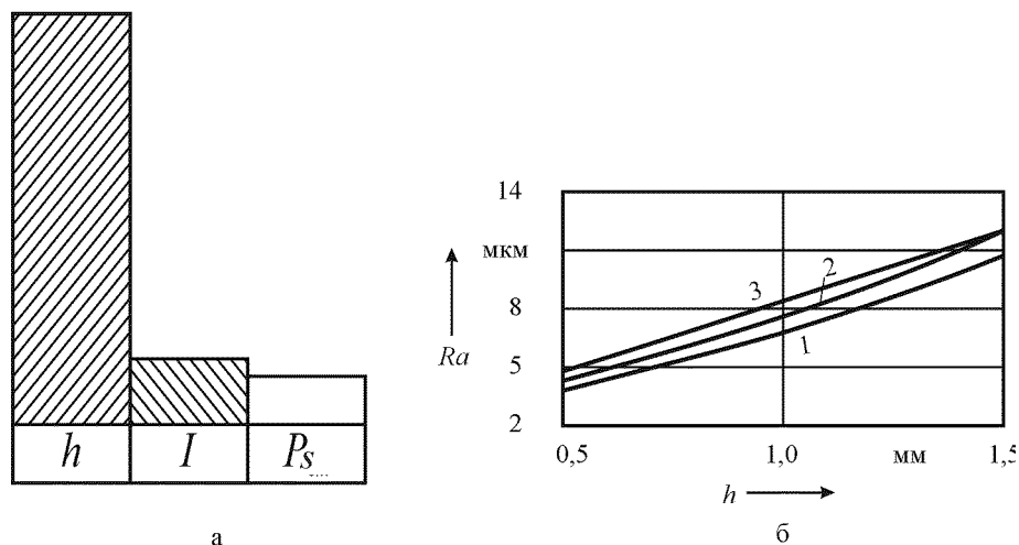
Рисунок 2 – Степень впливу факторів на шорсткість поверхні Ra (а) та залежність Ra від h та P_s ( I=100 А) (б)
