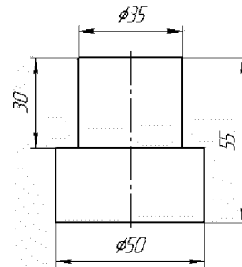
Рисунок 3 – Ступінчастий пуансон
