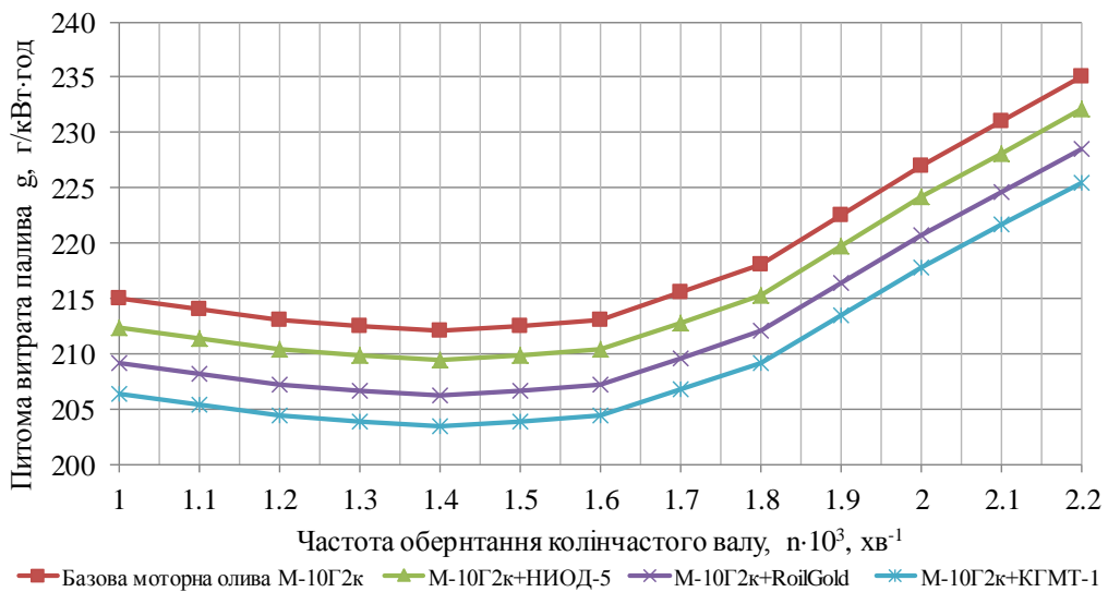
Рисунок 5 – Зовнішня швидкісна характеристика дизеля ЯМЗ-240 зі свіжою моторною оливою М-10Г 2 к та оливою з присадками НИОД-5, RoilGold і КГМТ-1: а – крутний момент; б – потужність; в – питома витрата палива
